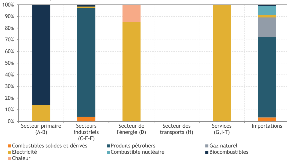
Graphique 4 Parts des produits énergétiques fournis par secteur agrégé et pour les importations En %, 2018
